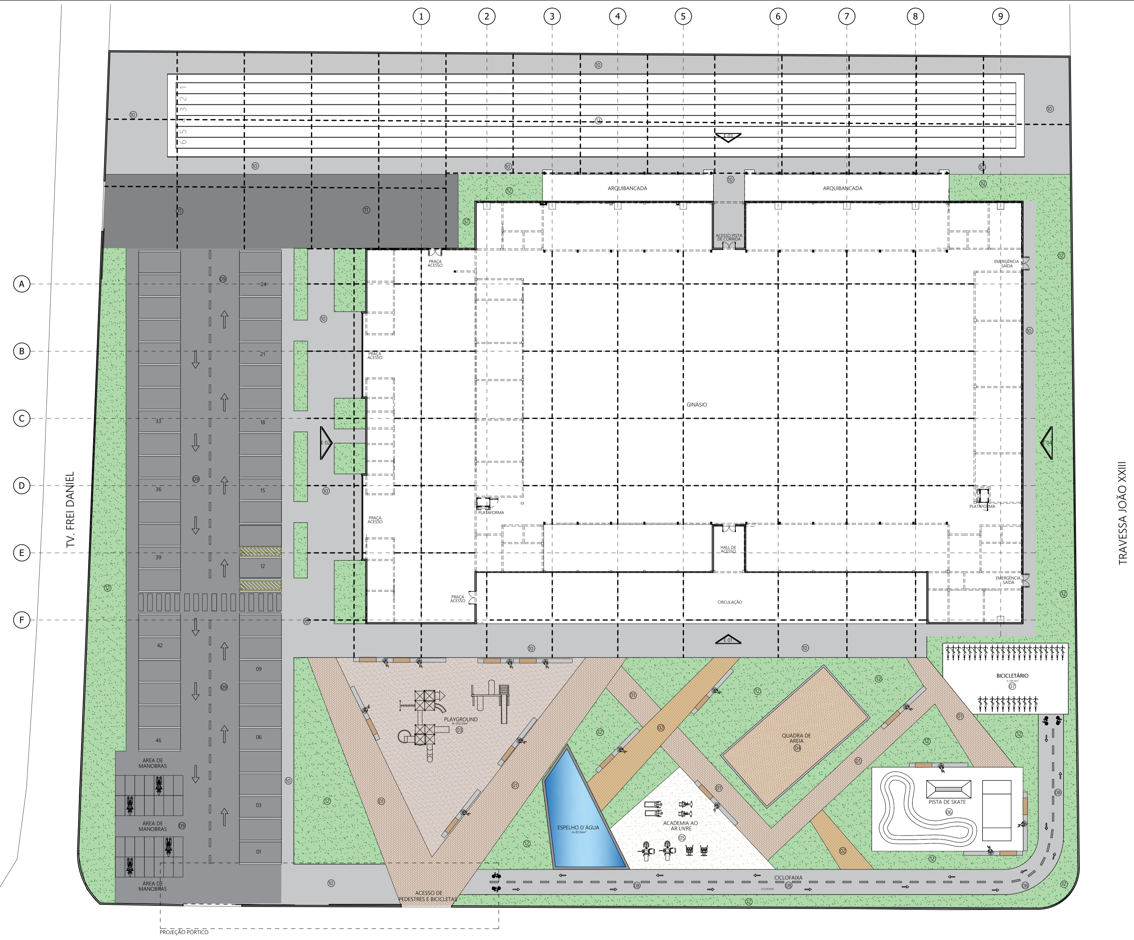
PLANTA BAIXA GERAL - TÉRREO
